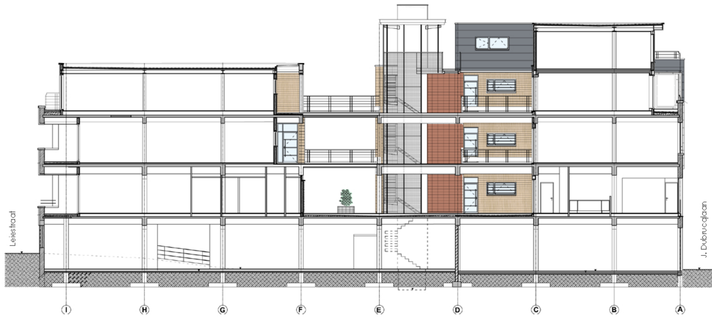
COUPE TRANSVERSALE B-B'
