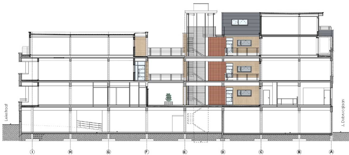
DWARSSNEDE B-B'
